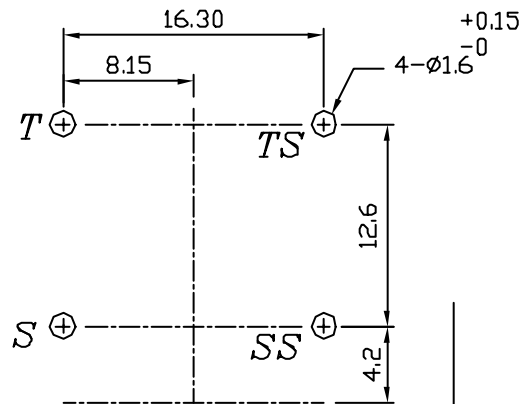
P.C.B LAYOUT(±0.1) (BOTTOM VIEW)
